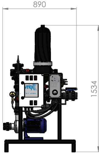
Ön Görünüş
