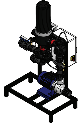
İzometrik Görünüş
